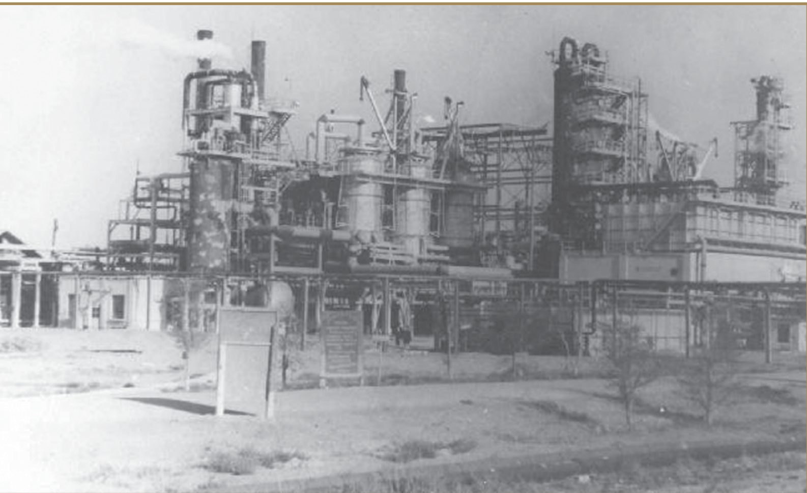
Гудри каталитикалық крекингінің қондырғысы Установка каталитического крекинга Гудри Goodry Catalytic Cracker Unit
