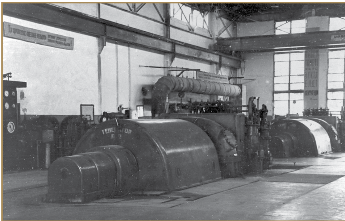
ЖЭО турбиналық залы Турбинный зал ТЭЦ Turbine room of Central heating and power plant
