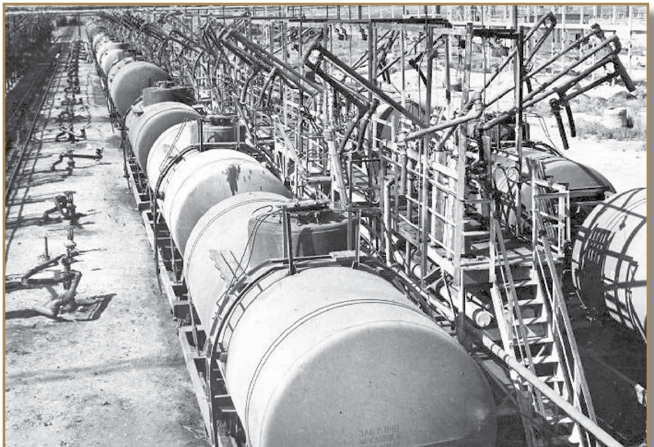
Мұнай өнімдерін құятын бірінші эстакада Первая эстакада налива нефтепро- дуктов First discharge rack
