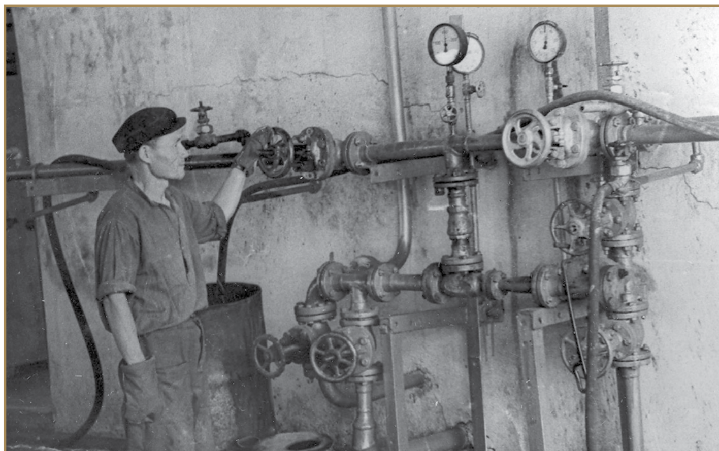
Тауар-шикізат цехының этил араластыру бөлмесі Этилосмесительная товарно-сырьевого цеха Ethyl Mixing Unit of the Raw Materials Shop
