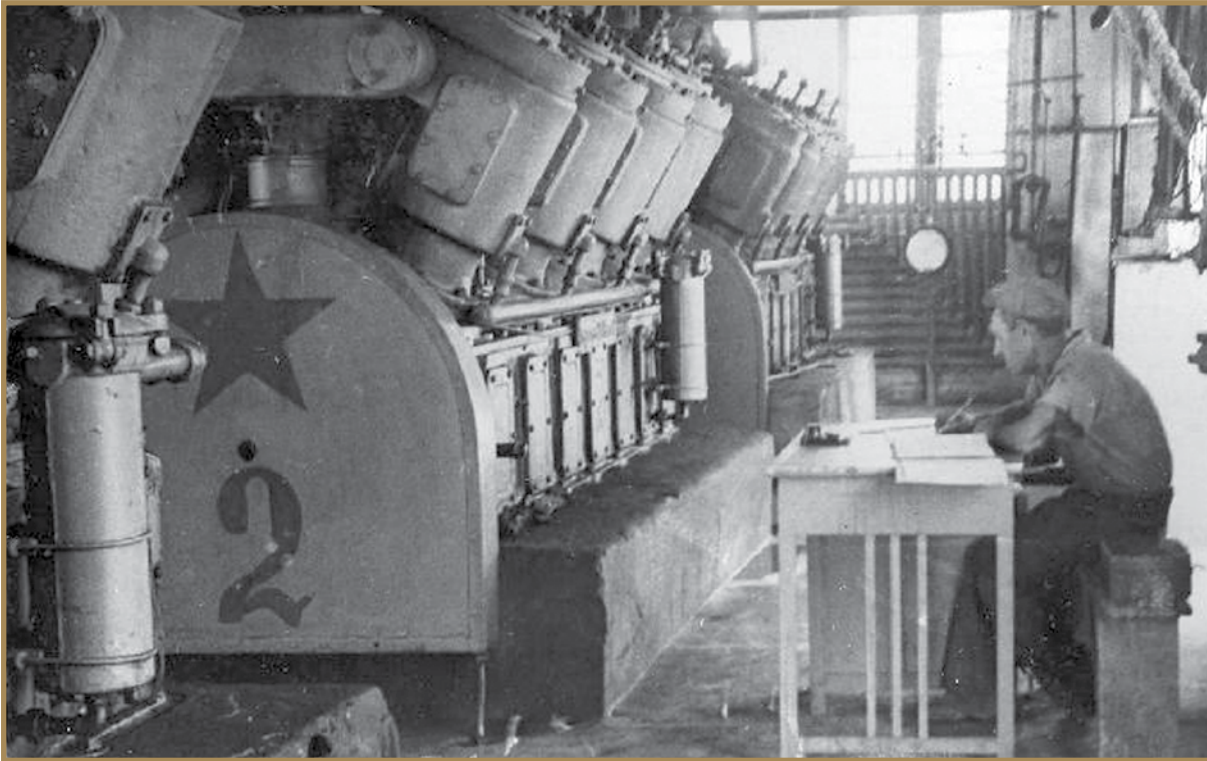
Күкірт қышқылын алкилдейтін қондырғының аммиакты компрессорлық станциясы Аммиачная компрессорная установки серно- кислотного алки- лирования Ammonium Compressor Facility of Sulfuric Acid Alkylation Unit
